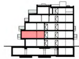
SCHNITT
