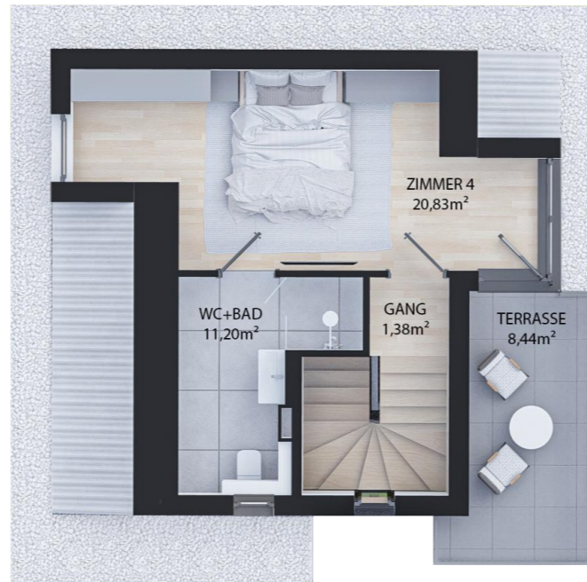
DACHGESCHOSS WNFL 33,41m 2
